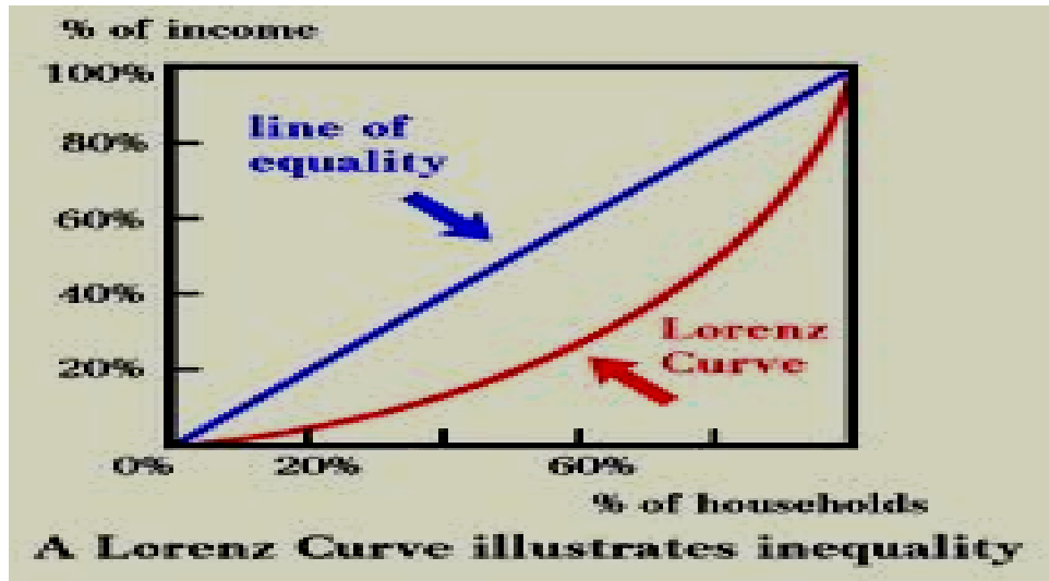
लॉरेन्स वक्र, भारत
